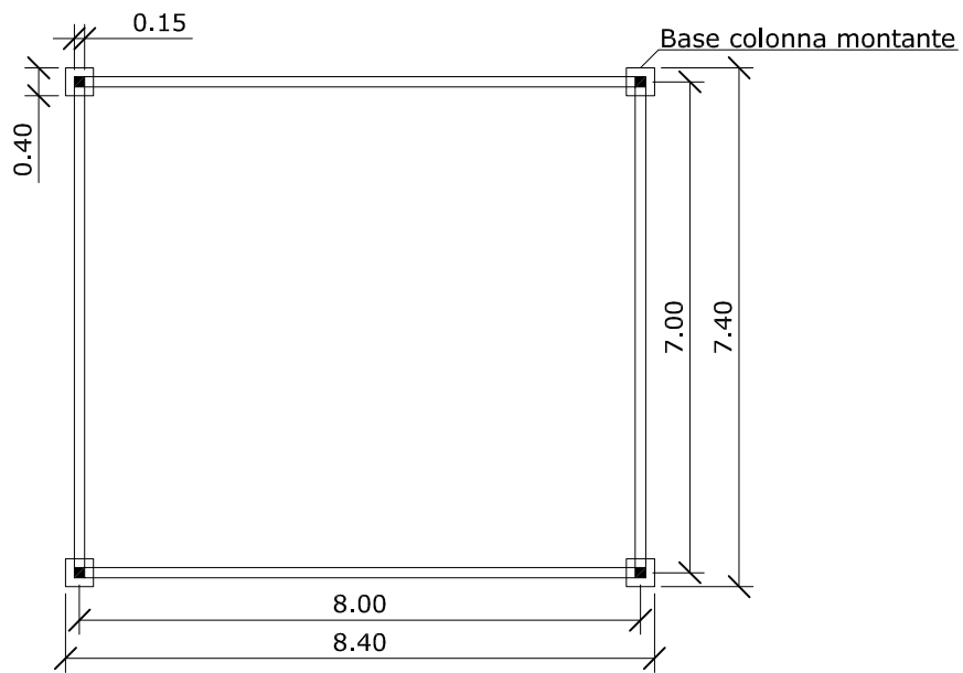
- PIANTA
