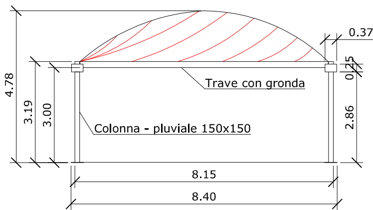
- PROSPETTO
